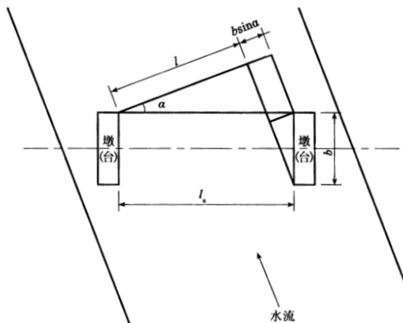
图3.2.3 墩（台）边缘净距计算简图
