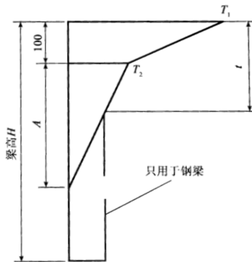
图 4.3.12 竖向梯度温度 (尺寸单位: mm)
