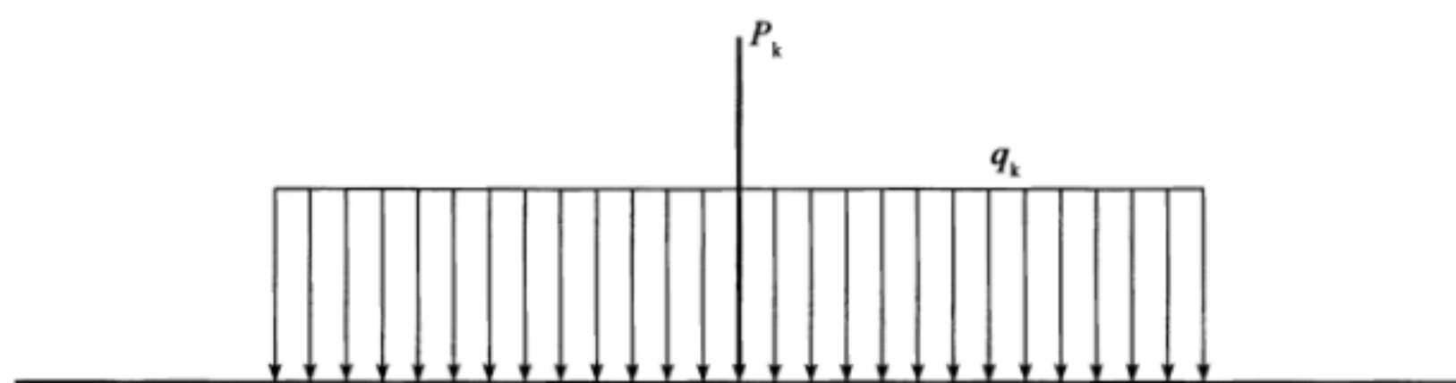
图 4.3.1-1 车道荷载
