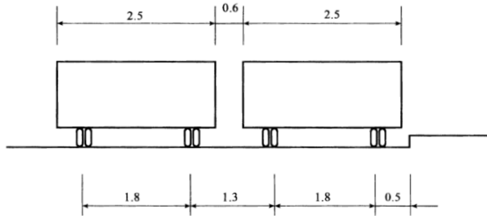
图 4.3.1-3 车辆荷载横向布置 (尺寸单位: m)
