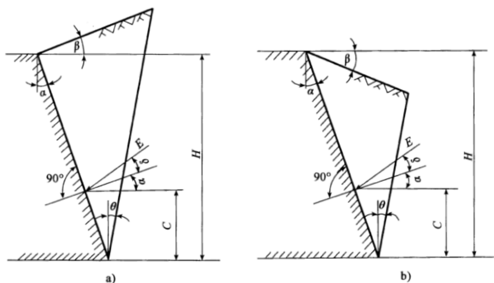
图 4.2.3-1 主动土压力图
