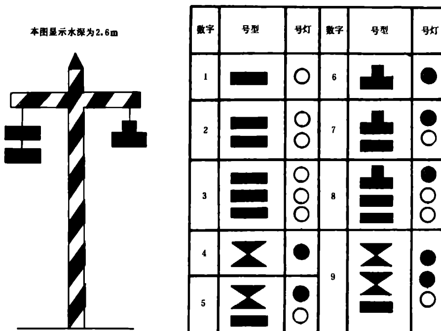
图 16 水深信号标及水深信号
